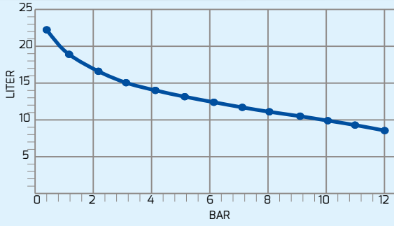
NOVA 25L/5B
