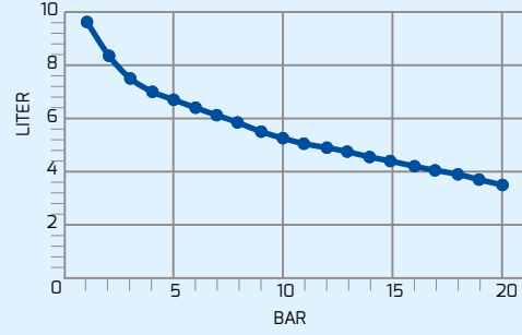
NOVA 3,5L/20B
