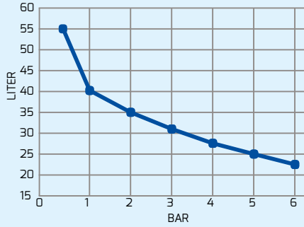
NOVA 25L/5B
